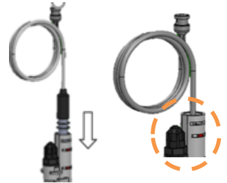
Une sonde 100% protégée par le tube du Porte Sonde
