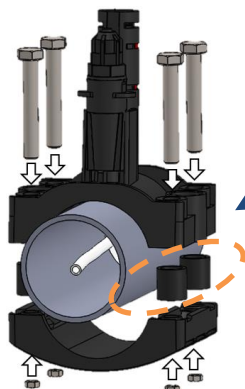
Tuyau DN50 ou DN63
